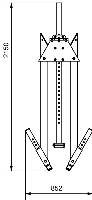
Seitengestell, geklappt
